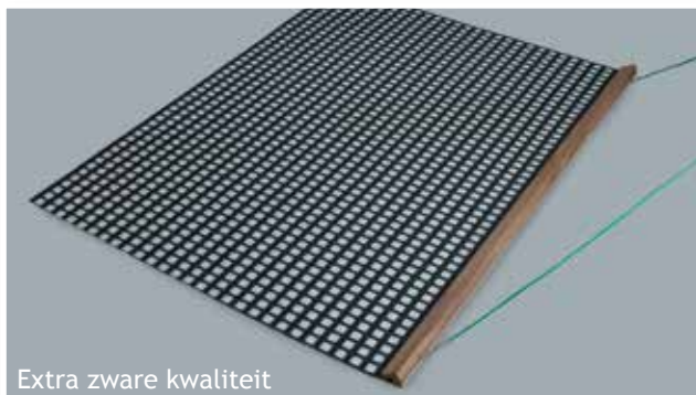
Enkel sleepnet "Speciaal". Houten trekbal met sleepnet en trekkoord. Werkbreedte 200 cm en lengte net 150 cm. Art.nr.41030 per stuk
