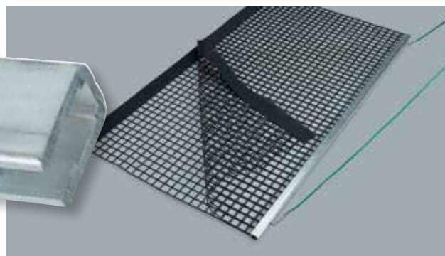
Dubbel sleepnet met aluminium trekbal. Aluminium trekbal met sleepnet en trekkoord. Werkbreedte 200 cm en lengte net 115 cm. Art.nr.41010 per stuk
